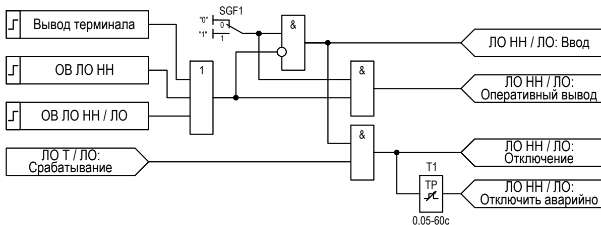
Рисунок 2.17 – Функциональная схема «ЛО»
