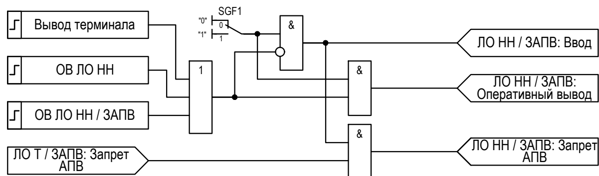
Рисунок 2.18 – Функциональная схема «Запрет АПВ»
