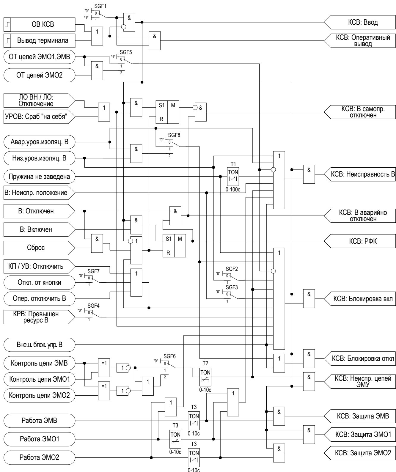
Рисунок 2.22 – Функциональная схема «КСВ»
