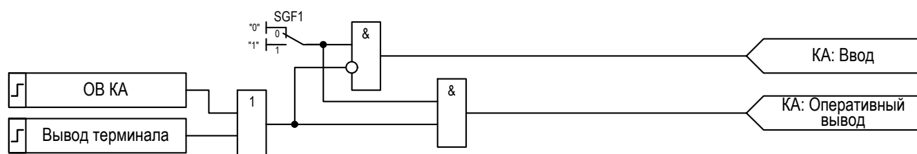
Рисунок 2.26 – Логика управления режимами функционального блока «КА»
