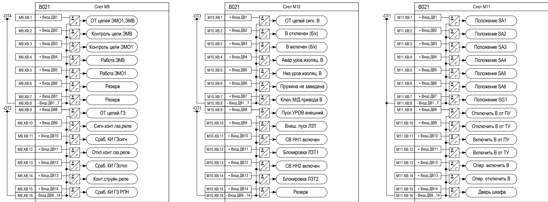
Рисунок Г.4 – Подключение дискретных входов и выходов к внутренним сигналам алгоритмов для блоков в слотах M9-M11
