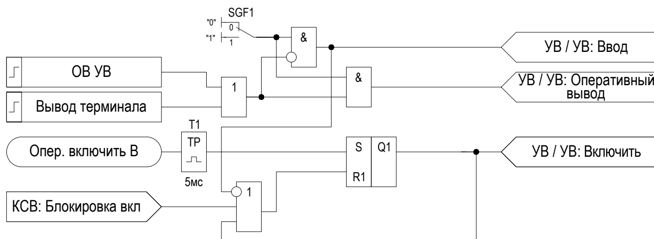
Рисунок 2.25 – Функциональная схема «УВ»
