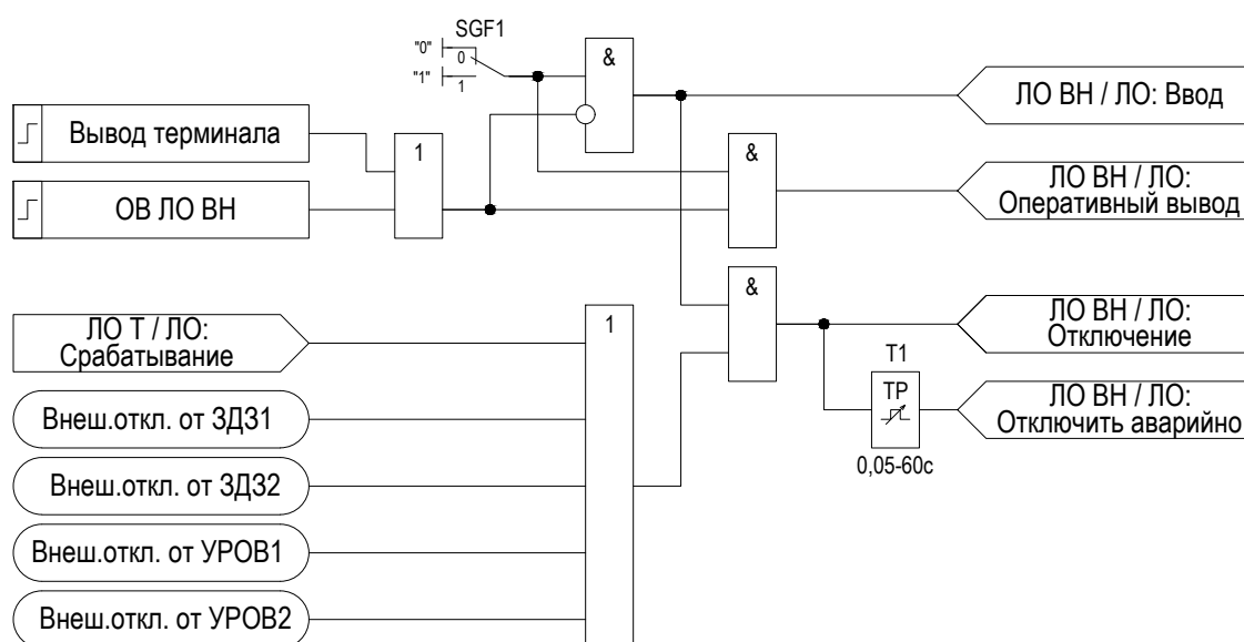
Рисунок 2.16 – Функциональная схема «ЛО»
