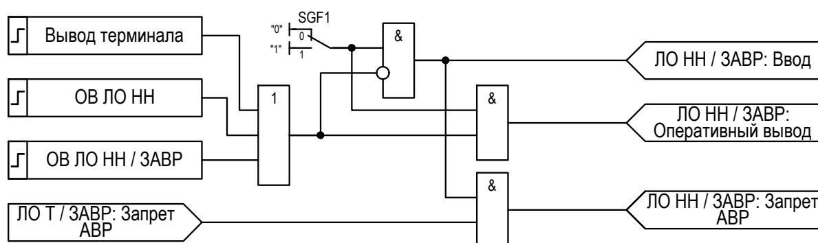
Рисунок 2.19 – Функциональная схема «Запрет АВР»
