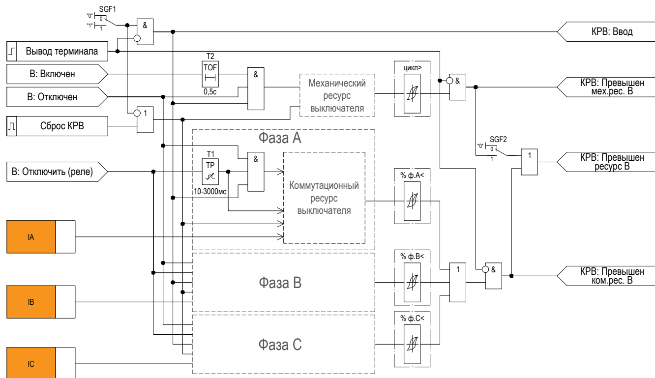
Рисунок 2.21 – Функциональная схема «КРВ»
