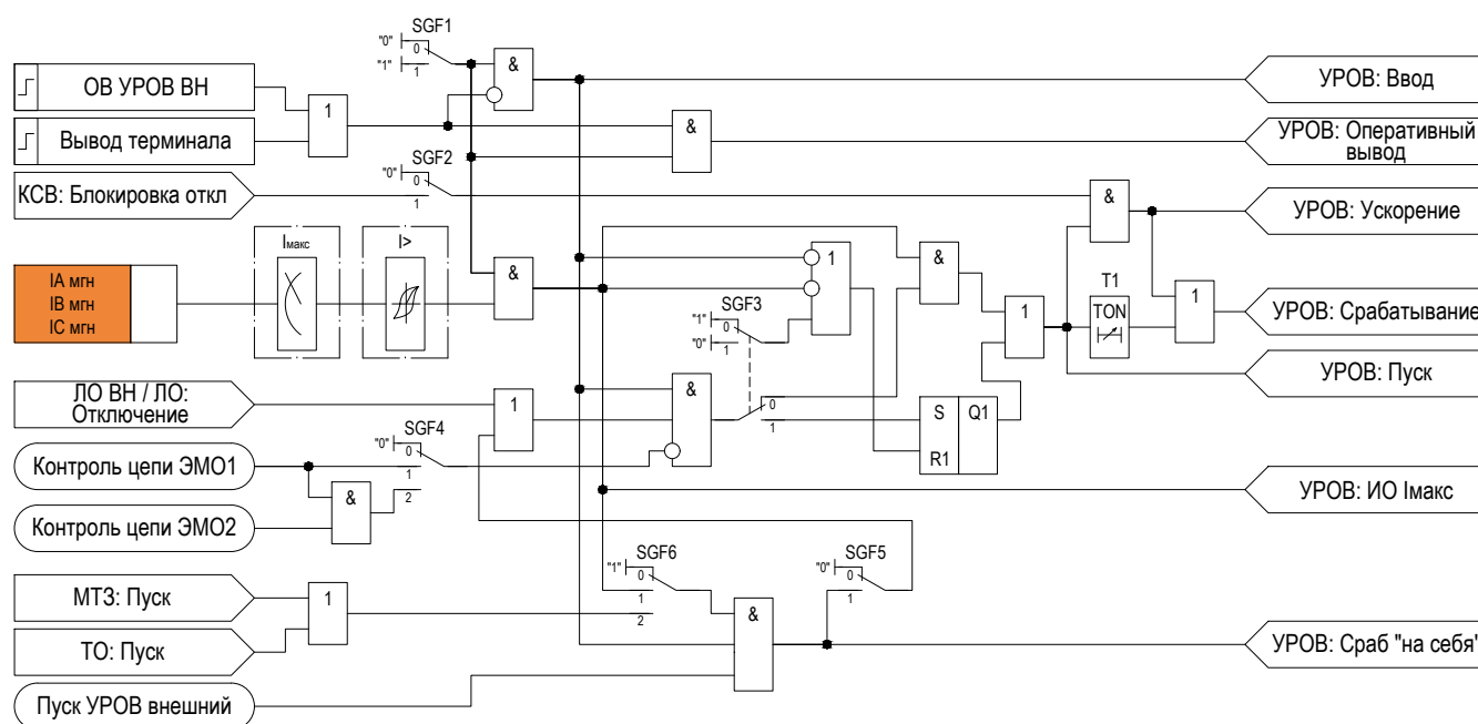
Рисунок 2.20 – Функциональная схема «УРОВ»
